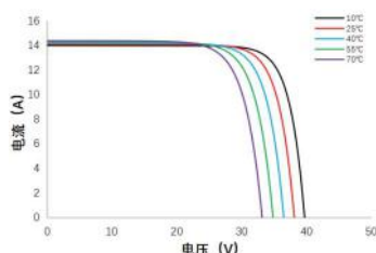
电流-电压曲线 SSA-48HD-445N
