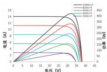
电流/功率-电压曲线 SSA-48HD-445N
