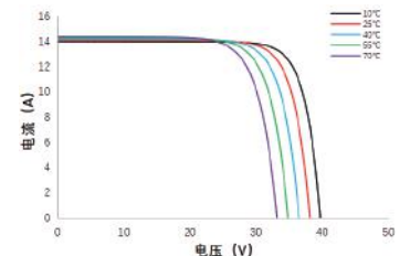
电流-电压曲线 SS8-54HDT-420N
