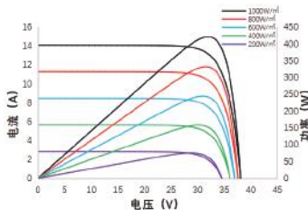
电流/功率-电压曲线 SS8-54HDT-420N
