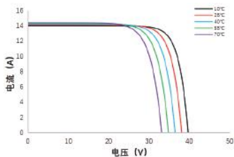
电流-电压曲线 SS8-54HD-420N
