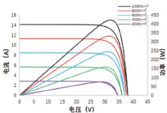
电流/功率-电压曲线 SS8-54HD-420N
