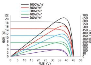
电流/功率-电压曲线 SS9-66HD-655M
