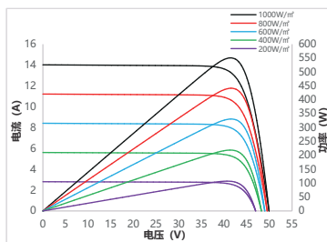
电流/功率-电压曲线 SS8-72HS -550M
