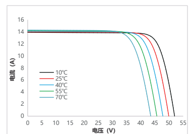
电流-电压曲线 SS8-72HS -550M
