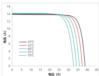
电流-电压曲线 SS8-54HS -410M
