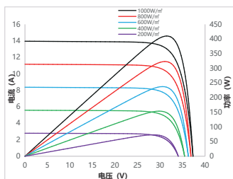
电流/功率-电压曲线 SS8-54HS -410M
