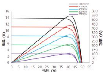
电流/功率-电压曲线 SS7-72HD-545M
