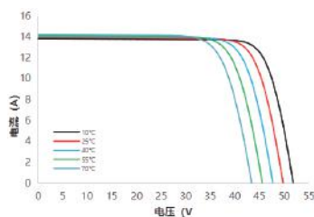
电流-电压曲线 SS7-72HD-545M
